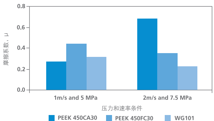
图 31：环块磨损试验测得的各种Vitrex材料的摩擦系数
