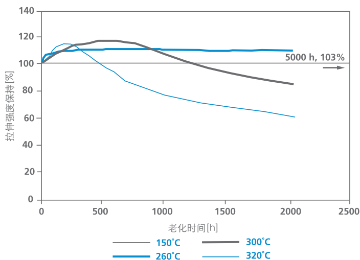
图 16 : 高温条件下未填充PEEK聚合材料的保留拉伸强度保持随时间变化的曲线图
