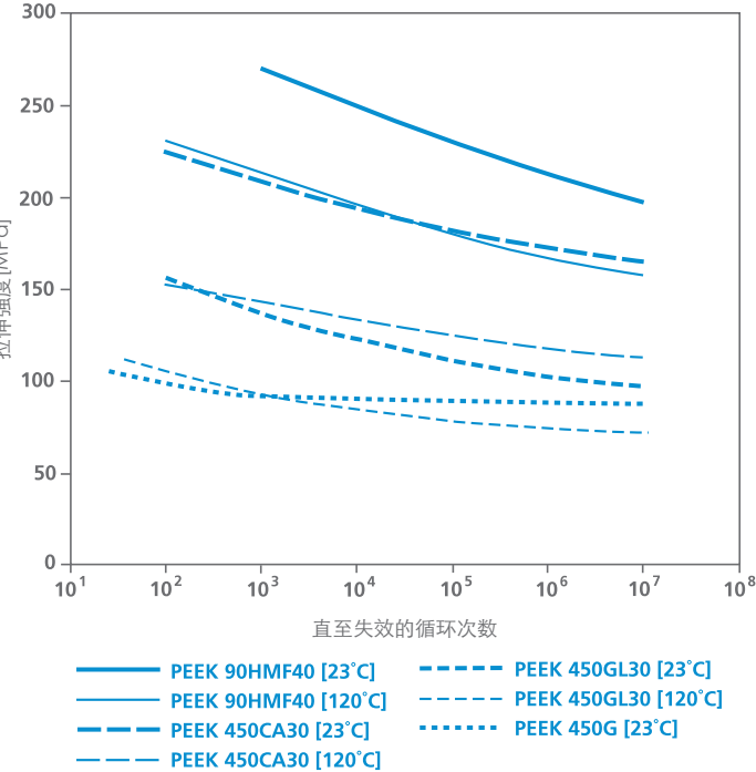
图 9 : 在5Hz、23℃和120℃条件下一组Victrex聚合材料的拉伸疲劳情况
