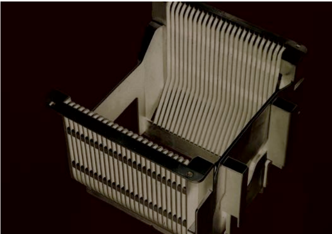
采用 VICTREX™ PEEK-ESD™ 聚合材料制作的晶圆卡匣能够控制静电电荷的耗散，保护晶圆免受损害，并通过减少和防止静电积聚保护晶圆免受由于静电吸引而造成的污染。
