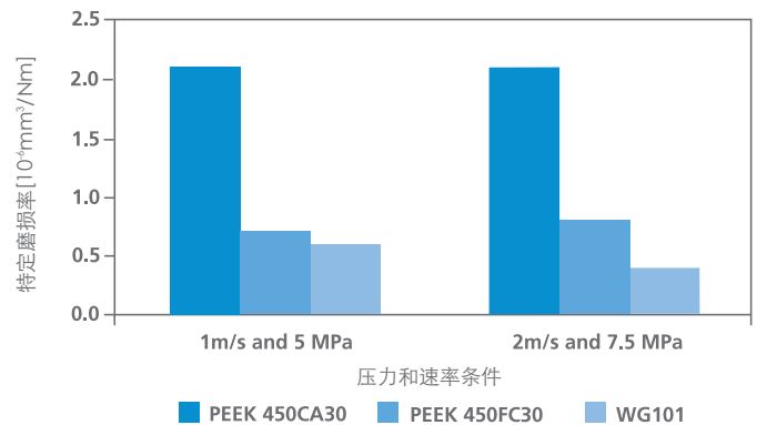
图 30：环块磨损试验测得的各种Vitrex材料的特定磨损率
